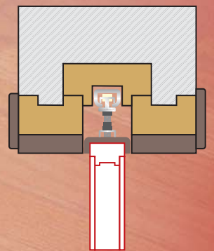
DETALLE SECCIÓN B
